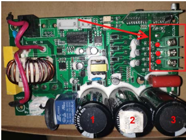
Рис 1. - Плата бесщеточного двигателя
