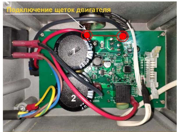
Рис 2. - Плата щеточного двигателя
